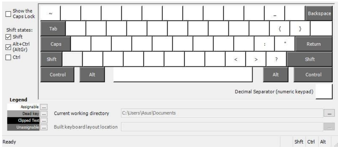
Shift + AltGr
